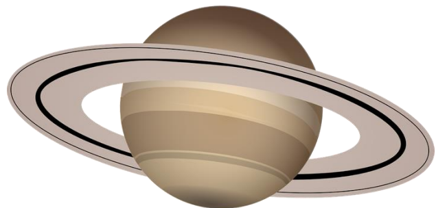
Une planète
