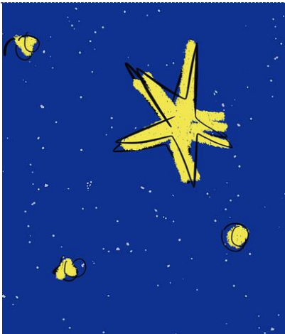
Une étoile
